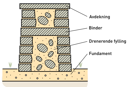
Fig 8.5 Tosidig mørtelmur av plater med avdekning.
