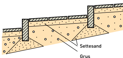
Fig 7.7 Terrengtrapp av plater med opptrinn av kantstein.
