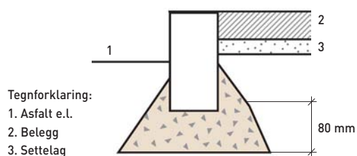
Fig 4.16 Kantstein på settelag av betong avsluttet mot belegg på settelag.
