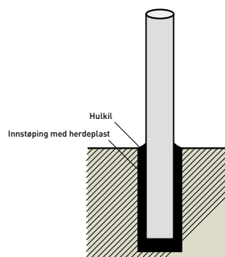
Fig 7.9 Innfesting av rekkverk i stein. Innstøping med herdeplast som trekkes opp til hulkiil.
