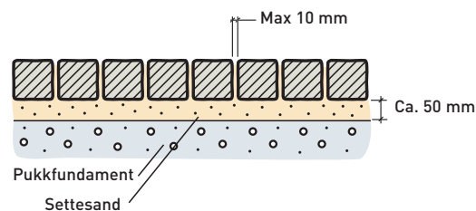
Fig 5.7 Typekonstruksjon.
