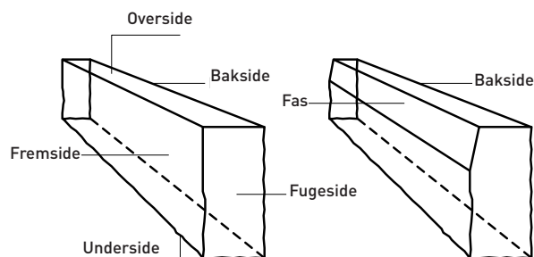
Fig 4.9 Benevning av kantsteinens ulike overflater.
