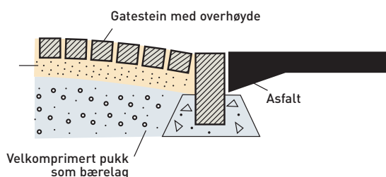
Fig 5.8 Markeringsfelt av gatestein med overhøyde.
