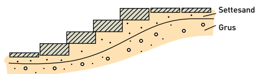
Fig 7.4 Terrengtrapp med massive trinn på grus og settesand.
