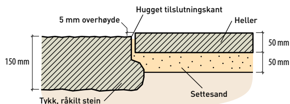
Fig 6.22 Overgang heller mot massiv stein.
