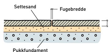
Fig 6.26 Setting av heller i sand på pukkfundament.
