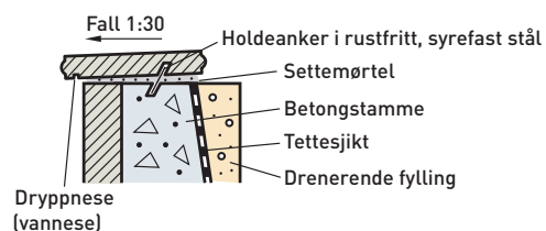
Fig 8.11 Støttemur med forblending og avdekning.
