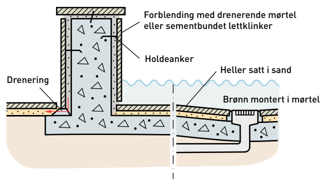
Fig 9.1 Oppbygging av fontene med steinplater på betongstamme.
