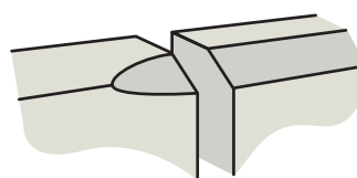
Fig 4.12 Avfasing i overgang mot faskantstein.
