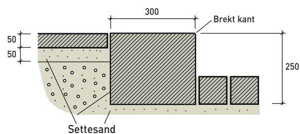
Fig 4.11 Platekantstein.
